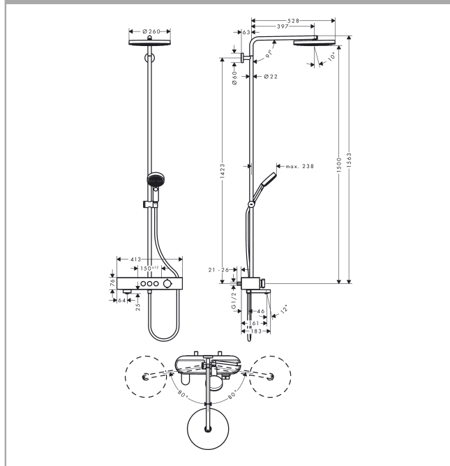
Plan coté
